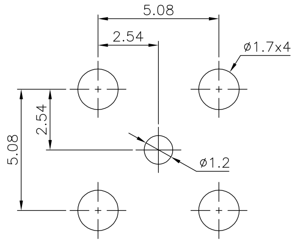
P.C.B. LAYOUT
